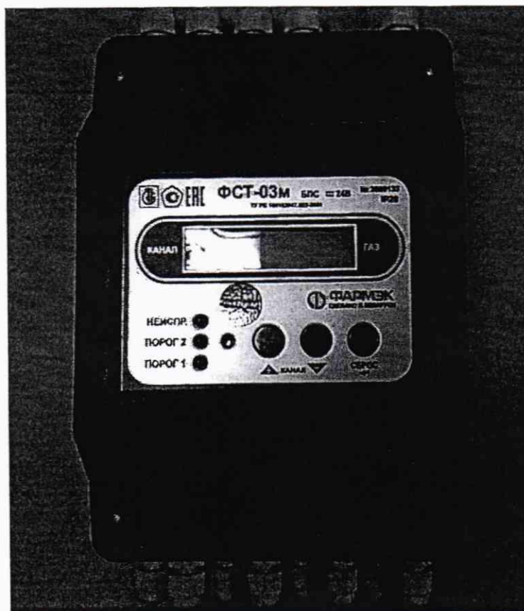
Рисунок 1а - Внешний вид газоанализатора ФСТ-03м с питанием от источника постоянного напряжения с номинальным значением 24 В.
