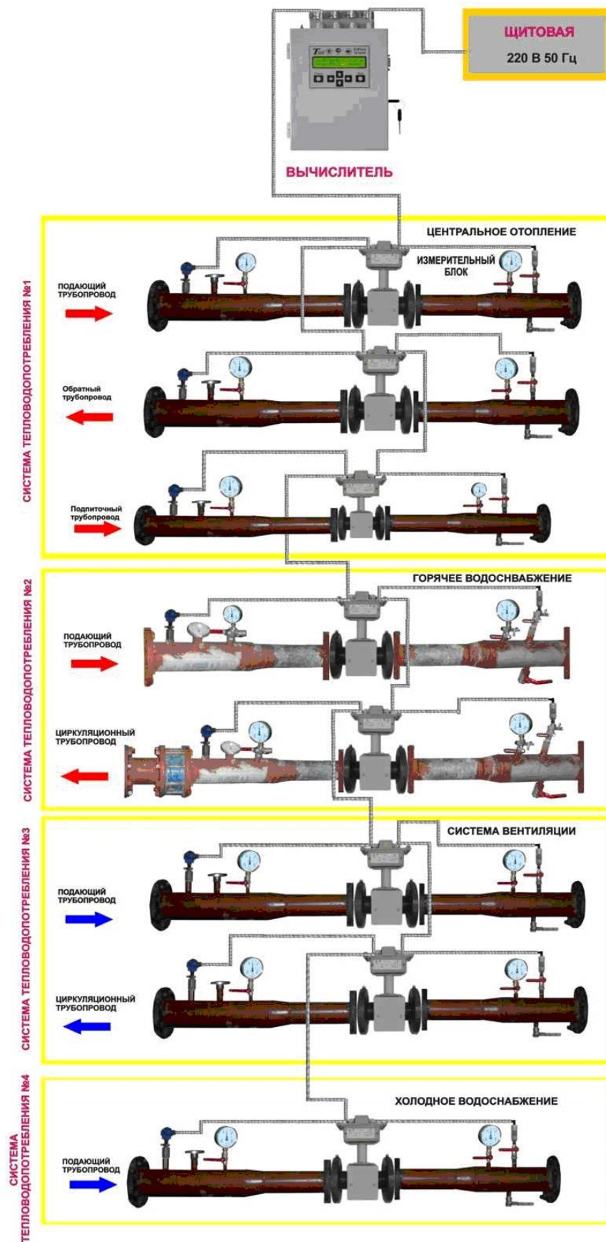
Рисунок Б.1 – схемы теплopotребления
