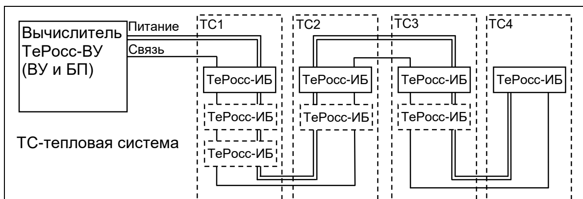
Рисунок 3.1 – Структурная схема прибора ТеРосс-ТМ
