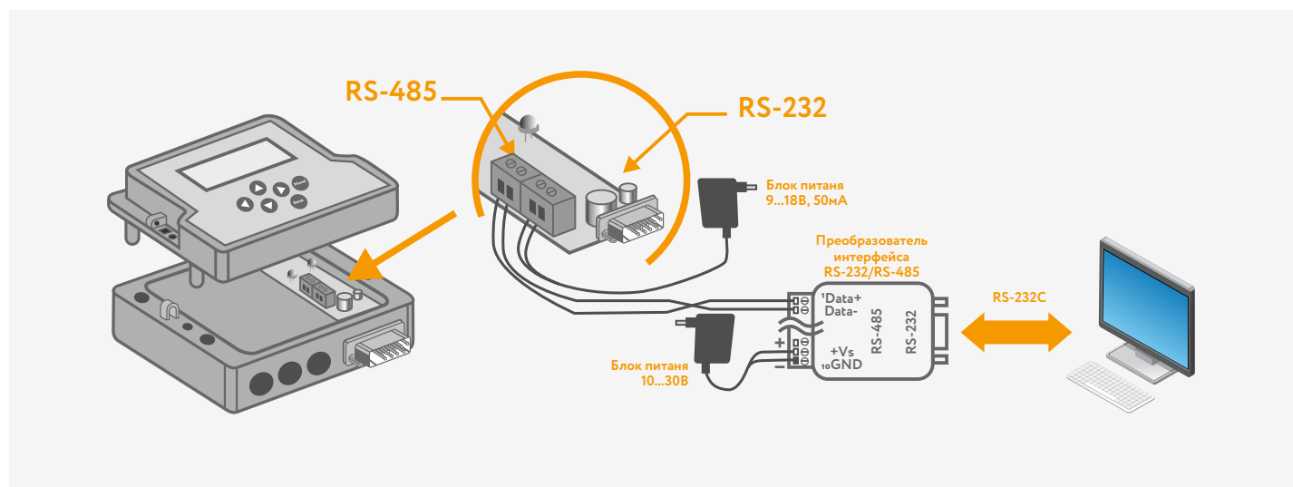
Рис. Д3 – Схема подключения адаптера интерфейса RS-485
