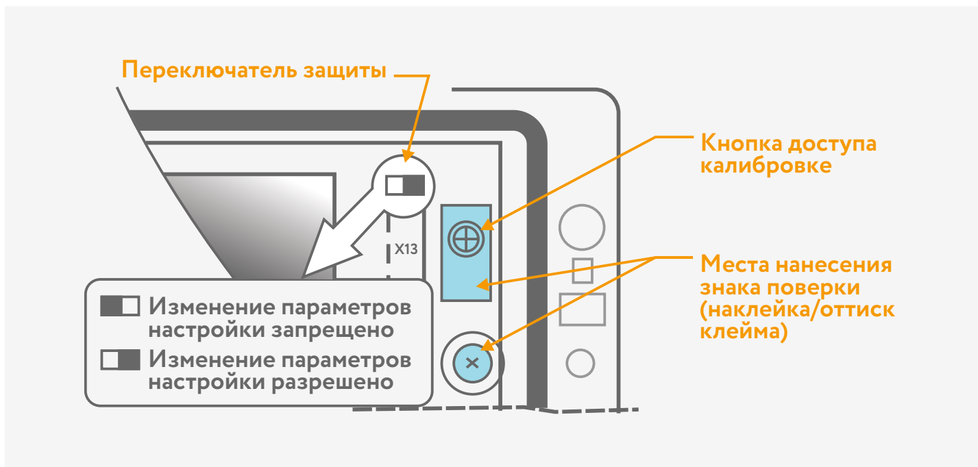
Рис. 1.2 – Места пломбирования поверителем
