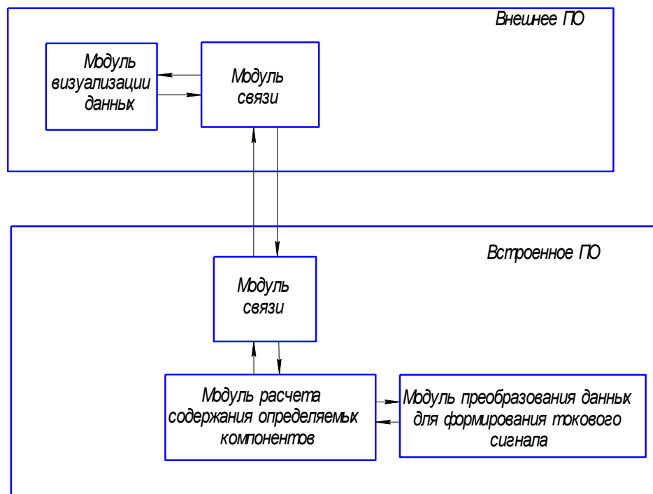
Рисунок 5 - Структура ПО.
