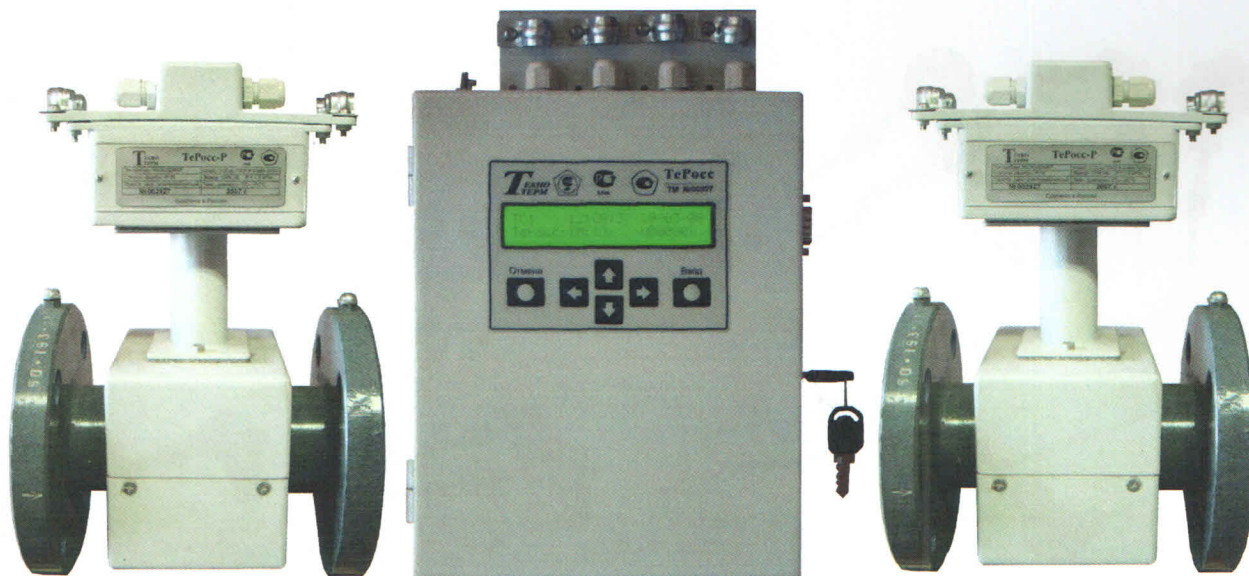
Рисунок 1 – Общий вид теплосчетчика TeRoss-ТМ с TeRoss-ВУ и TeRoss-ИБ в составе с ПРЭ
