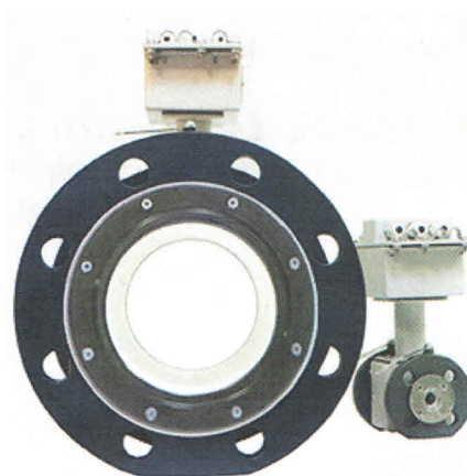
Рисунок 4.2 – Общий вид ПРЭ
